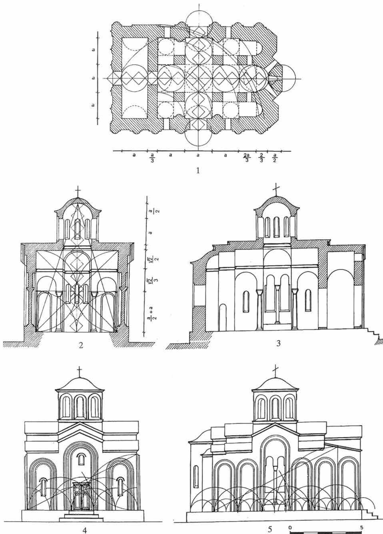
Обр. 1. Местността Бял бряг в Преслав, църква I: 1 - план на основите (метричен анализ); 2 - напречен разрез; 3 - надлъжен разрез; 4 - фасада-запад; 5 - фасада-север. Fig. 1. Byal Bryag locality near Preslav, Church I: 1 - plan of the substruction (metric analysis); 2 - cross-section; 3 - longitudinal section; 4 - façade-west; 5 - façade-north.
