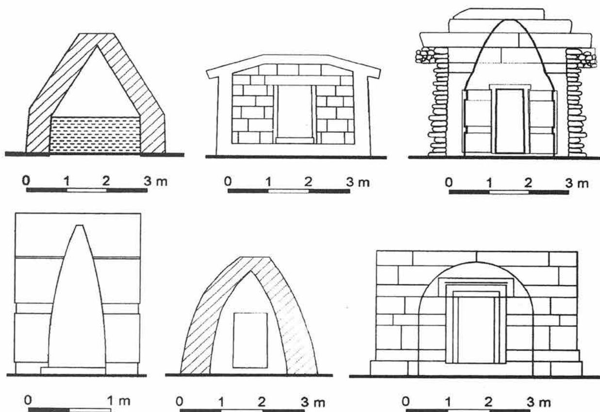
Обр. 16. Развитие от двускатно към полуцилиндрично покритие. Автор: Н. Тонков Fig. 16. Movement from gable to barrel-vaulted roof. Author: N. Tonkov
