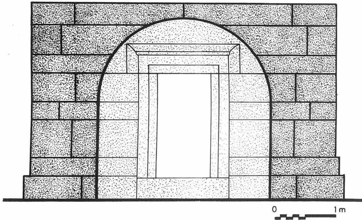
Обр. 1. Възстановка на преддверието и фасадата на храма в Славчова могила. Чертеж: Е. Крондева, С. Гощев.
