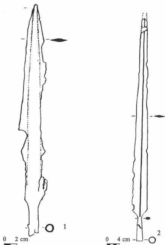
Обр. 2. Црънча. Графично изображение на железни копия от колективна находка Fig. 2. Tsrancha. Drawings of iron spearheads from a collective find
