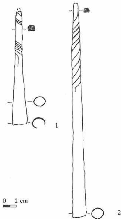
Обр. 3. Црънча. Графично изображение на железни накрайници за копие (сауротери) от колективна находка Fig. 3. Tsrancha. Drawings of iron spearpoints for (sauroters) from a collective find
