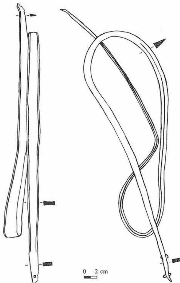
Обр. 5. Црънча. Графично изображение на железен меч-ромфея от колективна находка Fig. 5. Tsrancha. Drawing of an iron sward-rhomphaia from a collective find
