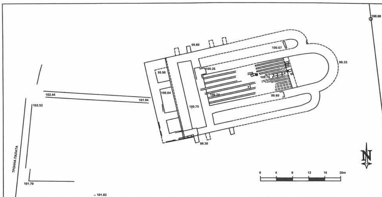
Обр. 2. Велики Преслав. План на владетелската църква Fig. 2. Plan of the royal church in Veliki Preslav
