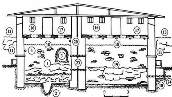
Обр. 6. Надлъжен разрез през щерни 1 и 2 - 2-ри етап - реконструкция (Е. Дерменджиев): 1. Щерна 1; 2. Утаител на щерна 1; 3. Каптажна ниша на щерна 1; 4. Водопровод 1; 10. Шахта; 11. Чешми; 13. Улица северно от щерните; 16. Етаж над щерните; 17. Отвори за черпене на вода; 18. Водно ниво; 19. Щерна 2; 20. Водопровод 2; 23. Свързващи тръби между щерна 1 и щерна 2; 24. Отточна тръба на щерна 2
