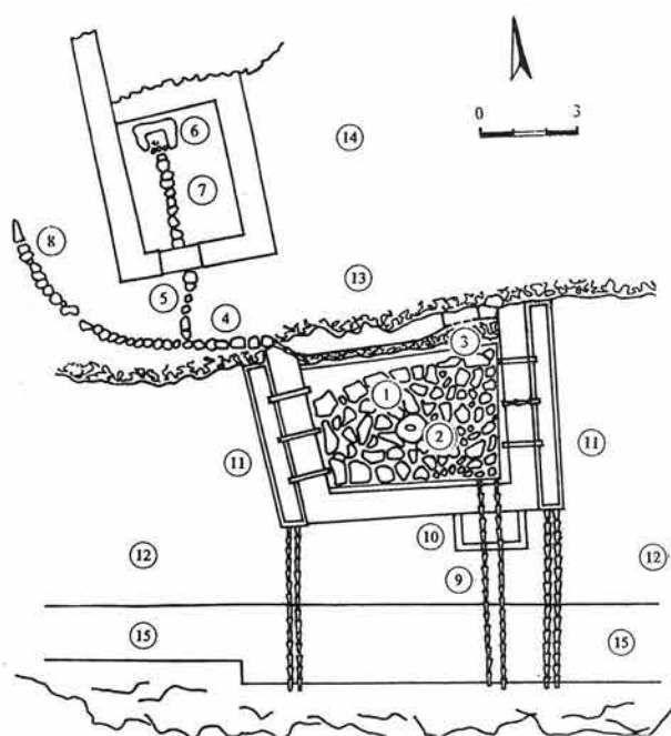
Обр. 3. План на водоснабдителните съоръжения при църква № 12 - I-ви етап - реконструкция (Е. Дерменджиев): 1. Щерна 1; 2. Утаител; 3. Каптаж на ниша; 4. Водопровод 1; 5. Водопровод 1А; 6. Каптаж на водопровод 1А; 7. Защитна сграда на каптаж 1А; 8. Водопровод 1Б; 9. Отточни тръби на щерна 1; 10. Шахта; 11. Чешми; 12. Улица край южната крепостна стена; 13. Улица северно от щерна 1; 14. Площад; 15. Южна крепостна стена
