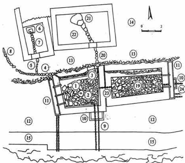
Обр. 5. План на водоснабдителните съоръжения при църква № 12 - 2-ри етап - реконструкция (Е. Дерменджиев): 1. Щерна 1; 2. Утаител на щерна 1; 3. Каптажна ниша на щерна 1; 4. Водопровод 1; 5. Водопровод 1А; 6. Каптаж на водопровод 1А; 7. Защитна сграда на каптаж 1А; 8. Водопровод 1Б; 9. Отточни тръби на щерна 1; 10. Шахта; 11. Чешми; 12. Улица край южната крепостна стена; 13. Улица северно от щерните; 14. Площад; 15. Южна крепостна стена; 19. Щерна 2; 20. Водопровод 2; 21. Каптаж на водопровод 2; 22. Защитна сграда на каптаж 2; 23. Свързващи тръби между щерна 1 и щерна 2; 24. Отточна тръба на щерна 2
