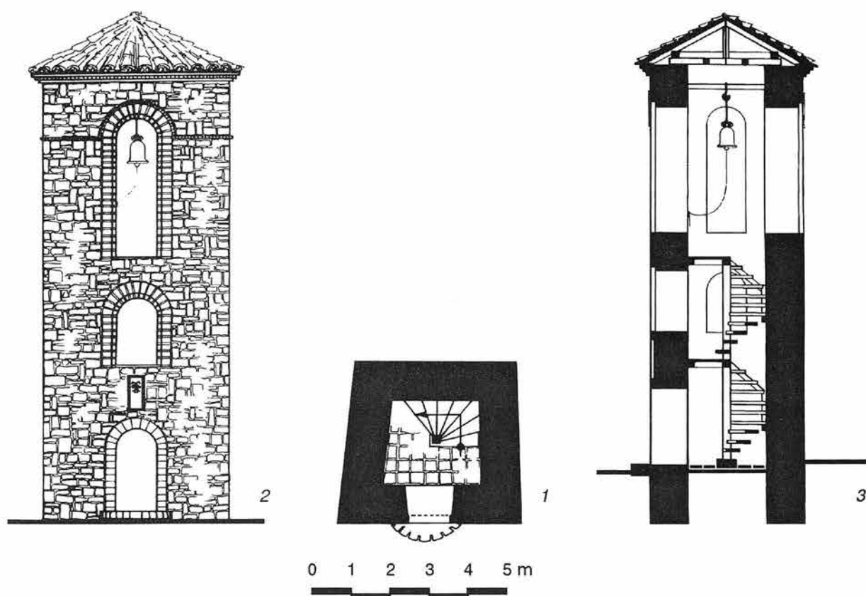
Обр. 4. Идеини реконструкции на средновековната кула-камбанария (по арх. Н. Тулешков). 1 - план; 2 - силует; 3 - вертикален разрез
