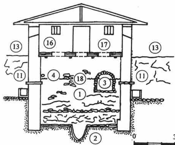
Обр. 4. Надлъжен разрез през щерна 1 - 1-ви етап - реконструкция (Е. Дерменджиев): 1. Щерна 1; 2. Утаител; 3. Каптажна ниша; 4. Водопровод 1; 11. Чешми; 12. Улица край южната крепостна стена; 13. Улица северно от щерна 1; 16. Етаж над щерната; 17. Отвори за черпене на вода; 18. Водно ниво Fig. 4. A longitudinal section through reservoir 1 (1st stage) - reconstruction of E. Dermendzhiev: 1 - reservoir 1; 2 - storage for sediments; 3 - catchment niche; 4 - water pipe 1; 11 - fountains; 12 - street along the south defensive wall; 13 - street to the north of reservoir 1; 16 - floor above the reservoir; 17 - openings for water drawing; 18 - water level
