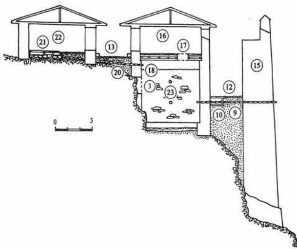
Обр. 7. Напречен разрез през щерна 1 - 2-ри етап - реконструкция (Е. Дерменджиев): 3. Каптажна ниша; 9. Отточни тръби на щерна 1; 10. Шахта; 12. Улица край южната крепостна стена; 13. Улица северно от щерните; 15. Южна крепостна стена; 16. Етаж над щерните; 17. Отвори за черпене на вода; 18. Водно ниво; 20. Водопровод 2; 21. Каптаж на водопровод 2; 22. Защитна сграда на каптаж 2; 23. Съвързащи тръби между щерна 1 и щерна 2 Fig. 7. Cross-section through reservoir 1 (2nd stage) - reconstruction of E. Dermendzhiev: 3 - catchment niche; 9 - draining pipes of reservoir 1; 10 - shaft; 12 - street along the south defensive wall; 13 - street to the north of the reservoirs; 15 - south defensive wall; 16 - floor above the reservoirs; 17 - openings for drawing water; 18 - water level; 20 - water pipe 2; 21 - catchment of water pipe 2; 22 - protective building above the catchment 2; 23 - pipes connecting reservoir 1 and reservoir 2
