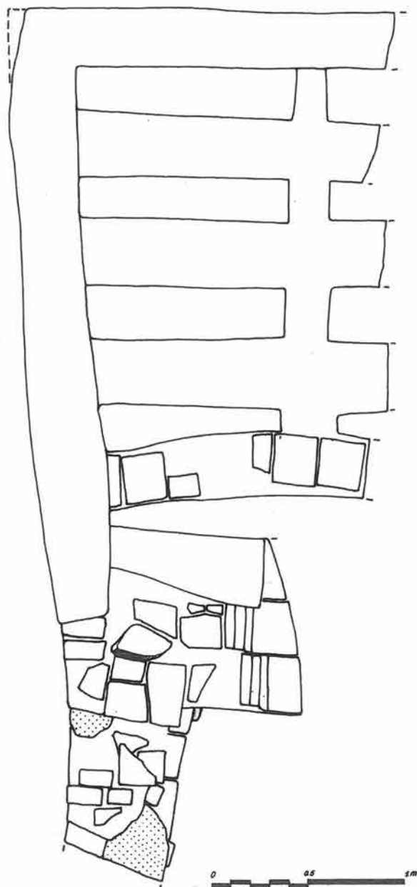
Обр. 4. Лозенец. План на запазена част от горната камера на пещта
