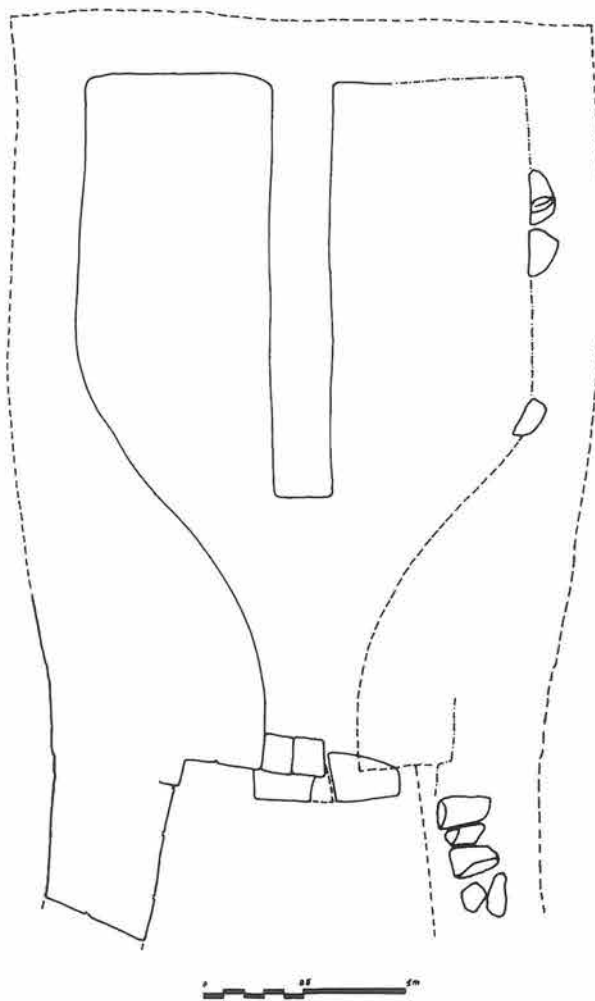
Обр. 3. Лозенец. План на долната камера на пещта Fig. 3. Lozenets. Plan of the lower chamber of the kiln
