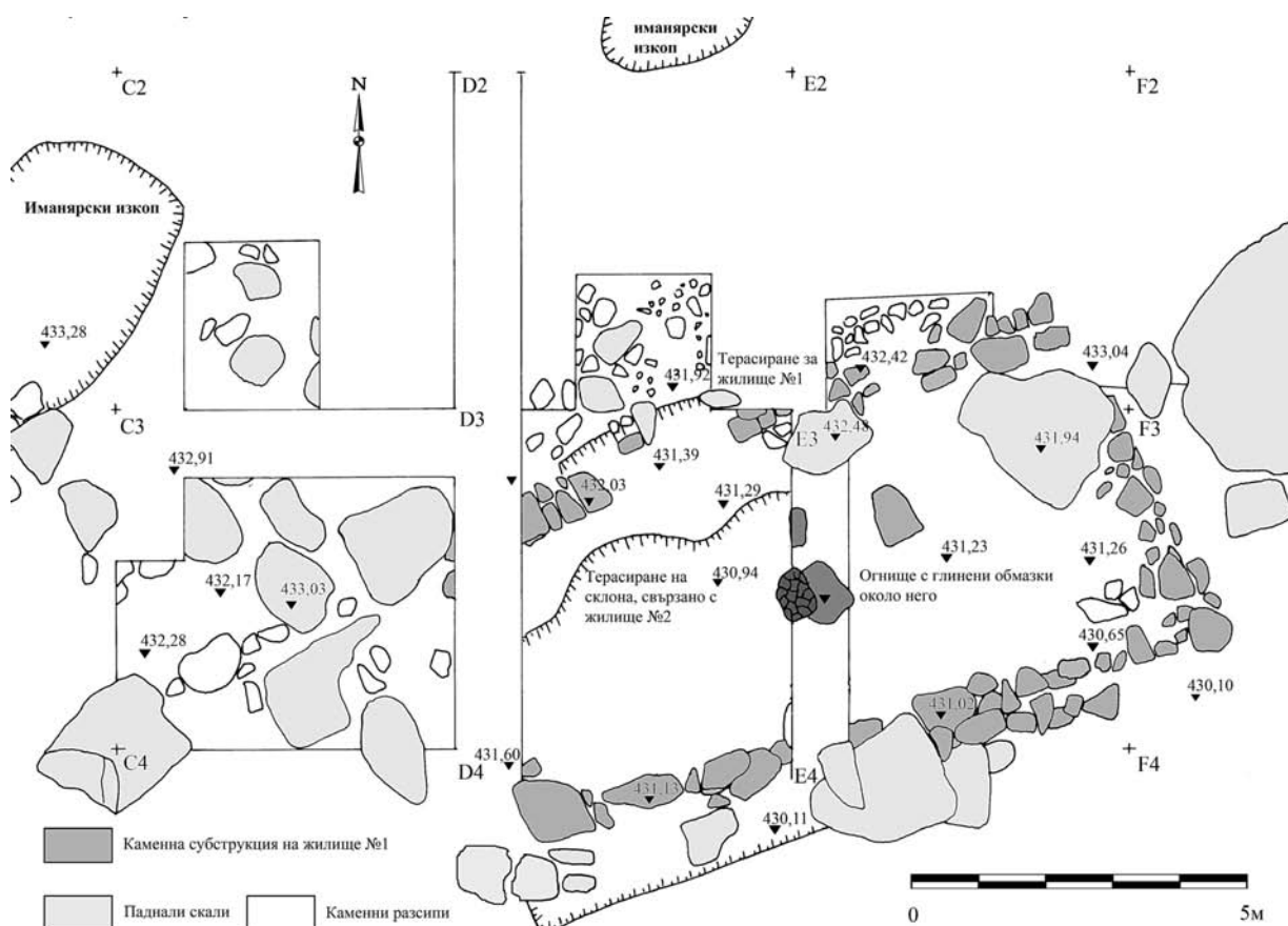
Обр. 5. Куш кая. Сектор I. Общ план на основите на жилище № 1 Fig. 5. Kush Kaya. Sector I. Sketch of the foundations of building No. 1
