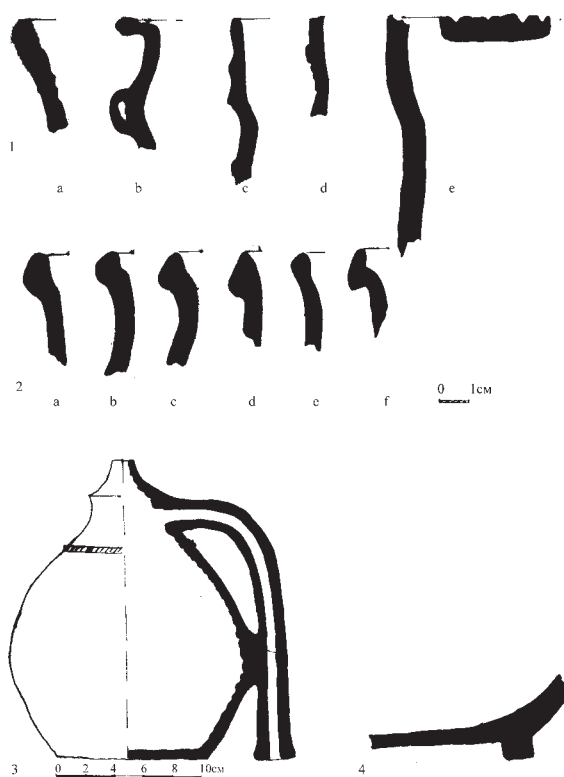
Обр. 14. Татул. Профили на средновековна керамика IX-XII в.: 1. Трапезна керамика със зелена глеч - а) купа, б) чаша, с - е) кани; 2. Кухненска керамика - а - ф) гърнета; 3. Кана с куха дръжка (аламбик) М:1:2; 4. Купа със златиста ангоба
