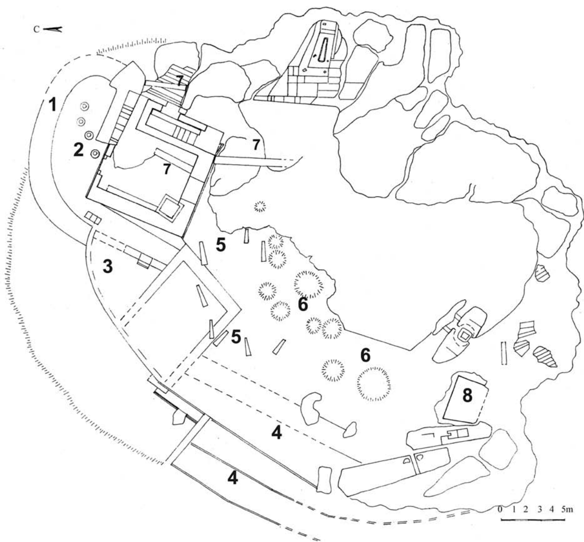
Обр. 8. Татул. План на извършените през средновековието реконструкции. Добавки от север на двора с питуосите от V-VI в., преустройства в сградите и по-късни (средновековни) терасирания от запад. Заснела: К. Симеонова. 1. Дъговиден зид пред сграда № 1 - ранновизантийска епоха (края на V в.); 2. Склад с питуоси (открити in situ) от V-VI в.; 3. Помещение между сгради № 1 и 2 с редица средновековни преустройства; 4. Средновековни подпорни зидове за терасиране на терена от запад; 5. Средновековният некропол на хълма Татул; 6. Средновековни боклучни ями; 7. Каменни зидове, преустрояващи пространството в и около сграда № 1 през средновековната епоха; 8. Сграда № 3 - късноримска / ранновизантийска епоха, т.нар. южна кула
