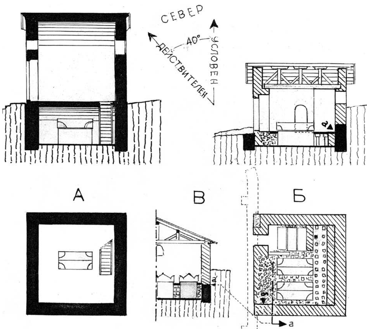
Обр. 1. Сердика. А План и разрез на хероона по оста изток-запад. Б План и разрез на временния мавзолей върху останките на криптата на хероона. В Разрез през западния край на южната стена на хероона и лежащата върху нея южна стена на мавзолея
