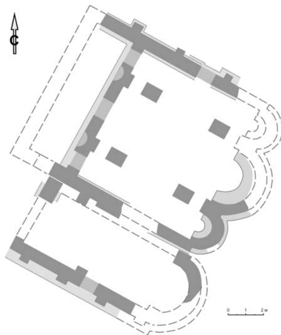
Обр. 3. Созопол. Примерна графична възстановка на храмовете (изработил: инж. А. Каменаров)
