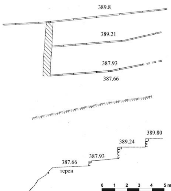
Обр. 9. Татул. Средновековни подпорни зидове за терасиране на пространството от запад. Заснела: К. Симеонова
