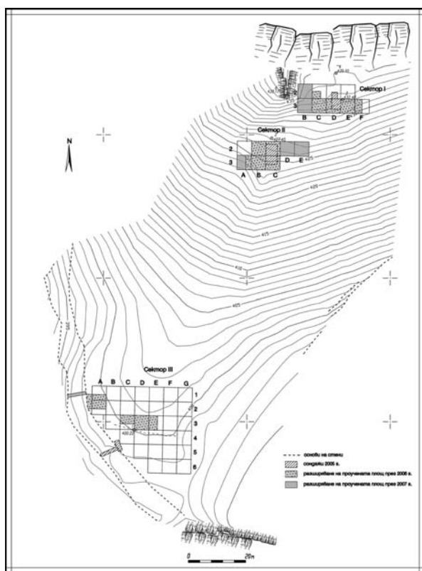
Обр. 3. Куш кая. Сектори I-III и напречни разрези на западната крепостна стена. Проучвания 2005-2007 г. Автор на заснемането Бистра Гяурова Fig. 3. Kush Kaya. Sectors I-III and cross-sections of the western fortress wall. Excavations 2005-2007. Drawn by Bistra Gyaurova
