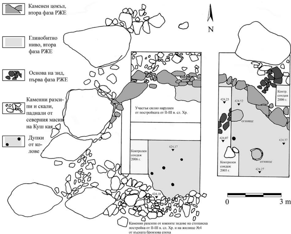
Обр. 15. Куш кая. Общ план на част от разкритите в Сектор II структури. Втора фаза на ранножелязната епоха
