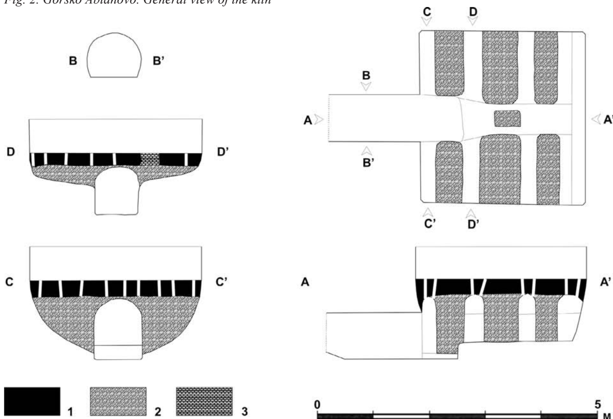
Обр. 3. Горско Абланово. Хоризонтален план на долната камера на пещта и вертикални разрези. Легенда: 1. Скара; 2. Елементи на носещата конструкция на скарата; 3. Деструкции Fig. 3. Gorsko Ablanovo. Horizontal plan of the lower chamber and vertical cross-sections. Key: 1 Grill; 2 Elements of the support construction of the grill; 3 Ruins
