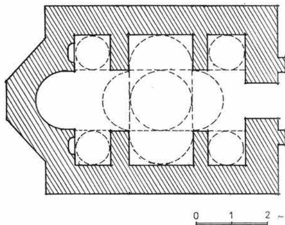
• Обр. 7. Пълна реконструкция на плана и фасадна перспектива по Г. Атанасов (първи вариант). Fig. 7. Reconstruction complete du plan et perspective de la facade d'après G. Atanasov (premiere variante)
