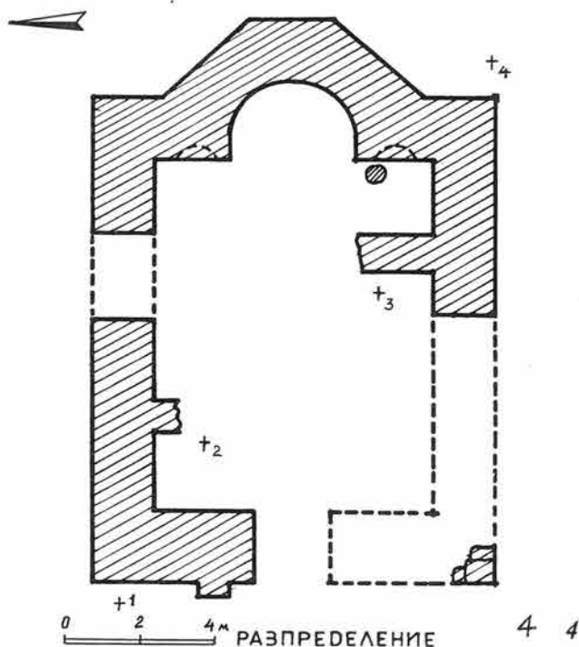
● Обр. 4. План на църква № 1 с отбелязани пастофории и гробове. Fig. 4. Plan de l'église No 1 avec indications de pastophores et de tombes
