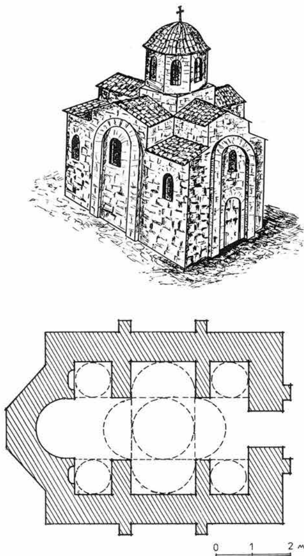
● Обр. 8. Пълна реконструкция на плана и фасада перспектива по Г. Атанасов (втори вариант). Fig. 7. Reconstruction complete du plan et perspective de la facade d'après G. Atanasov (deuxieme variante)
