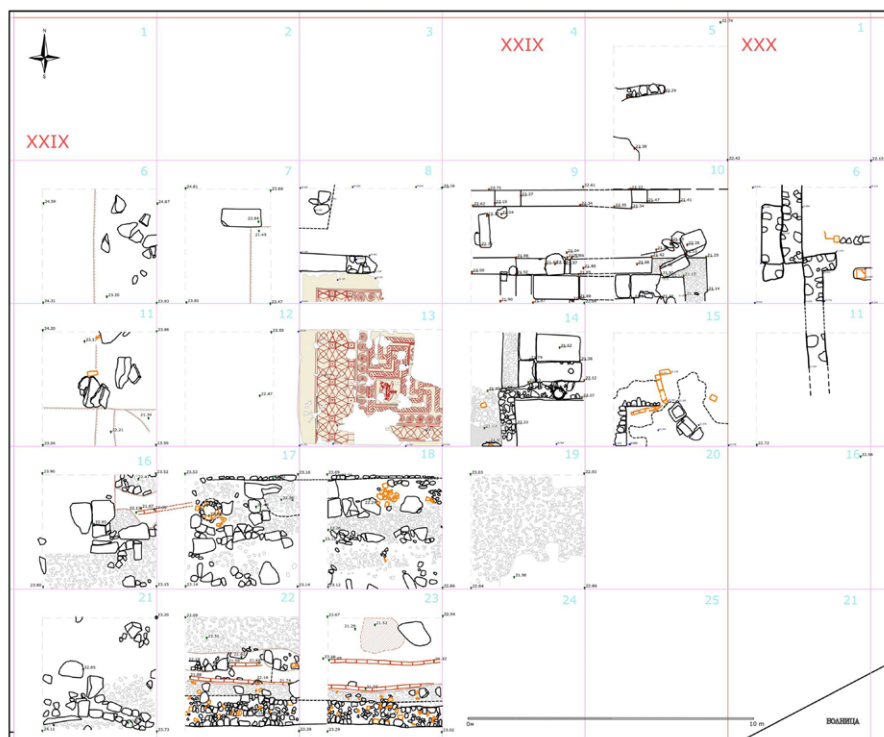
Обр. 2. Геодезическо и графично заснемане на проучвания сектор „Базилика“, Марцианопол/ис (Мартин Вълчев)
