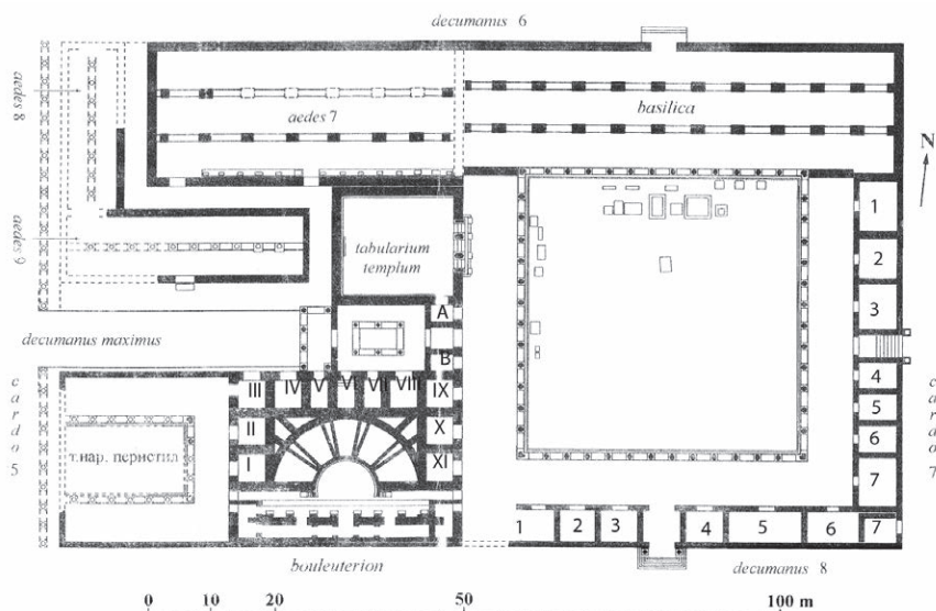
Обр. 2. План на форума на Никополис ад Иструм (по В. Динчев 2009, 72, обр. 2; Иванов, Иванов 1994 и с малки уточнения от автора).
