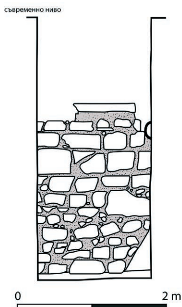
Обр. 3. Външно лице на крепостната стена по ул. „Седми септември“ № 17-19.
