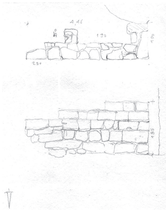
Обр. 6. Храмът на Зевс Хипердексиос. Северни основи – план и изглед от С (личен архив Л. Маринов).
