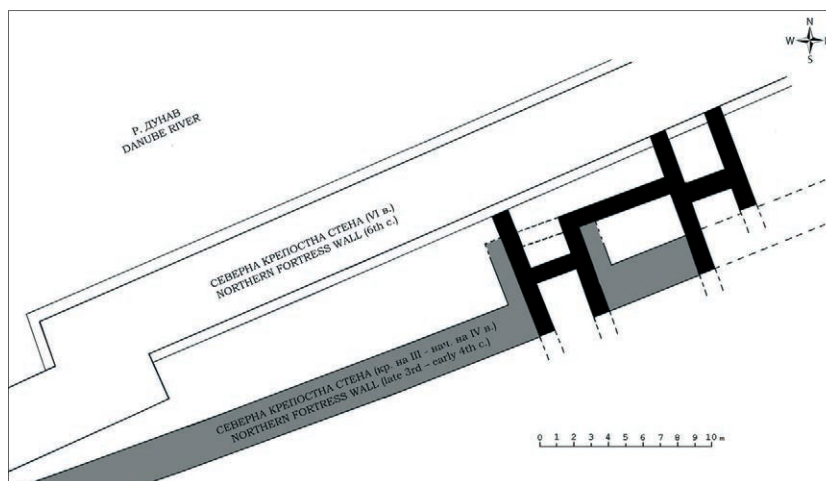
Обр. 4. План на северната крепостна стена с кула на ранния дунавски кастел от кр. на III – нач. на IV в.
