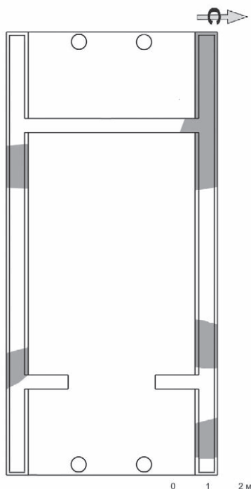
Обр. 11. Храмът на Зевс Хипердексиос (планова композиция и метрична реконструкция Х. Прешленов; графично представяне А. Каменаров).
