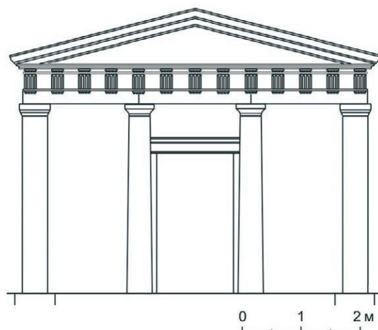
Обр. 13. Храмът на Зевс Хипердексиос – фасада (реконструкция Х. Прешленов; графично представяне А. Каменаров).
