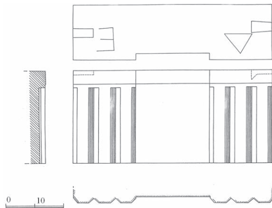
Обр. 12. Фризов блок от храма на Зевс Хипердексиос (рисунка Д. Стоянова).
